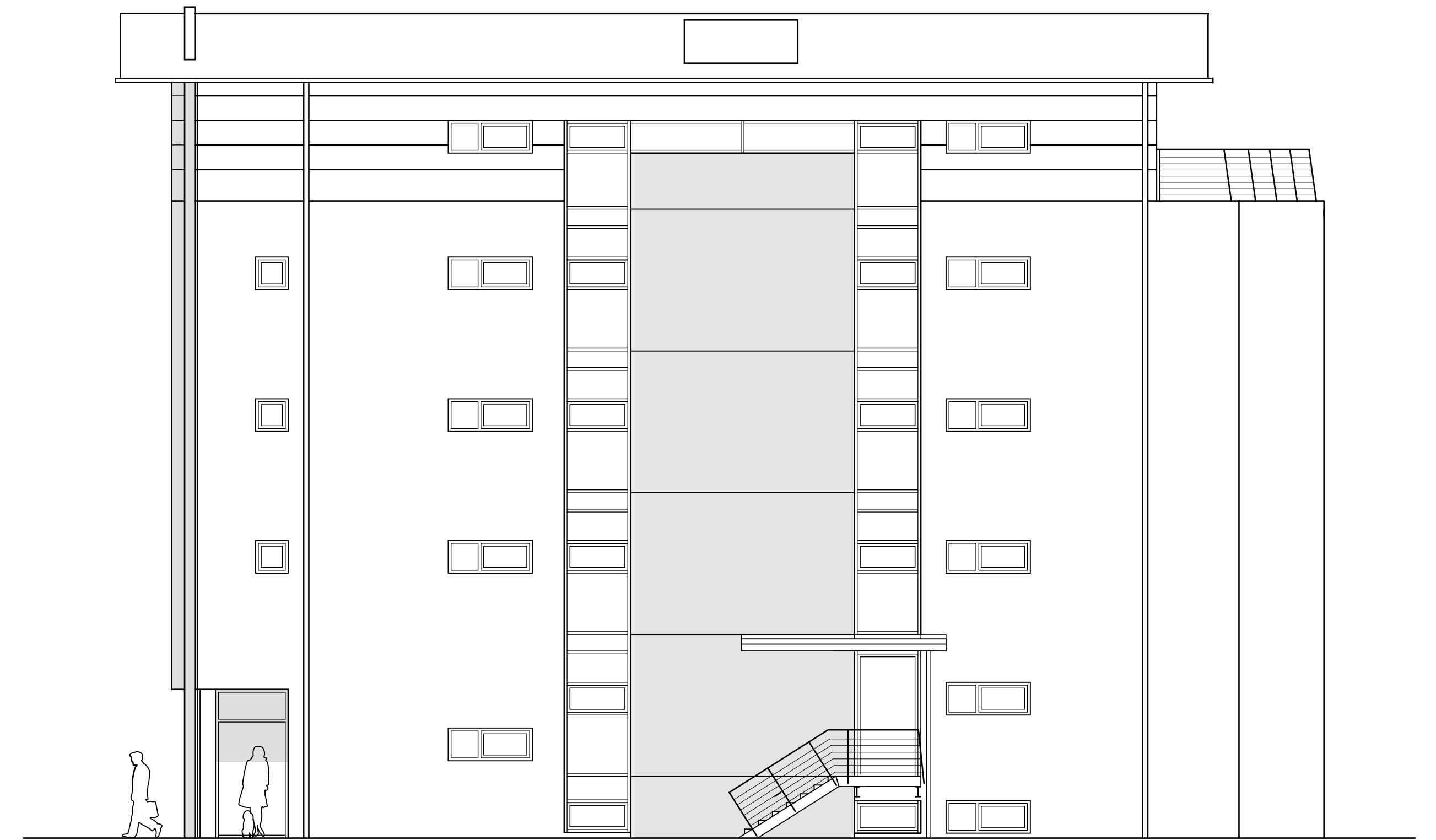
ANSICHT WEST
